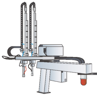
機器手臂
