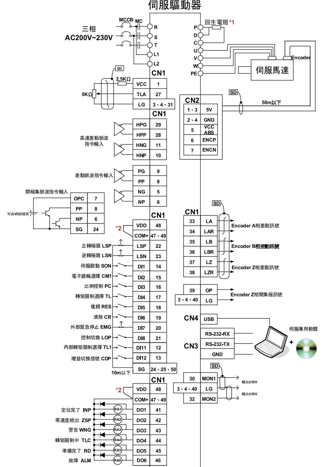
■ Pt Mode: 位置控制模式接線示意圖
