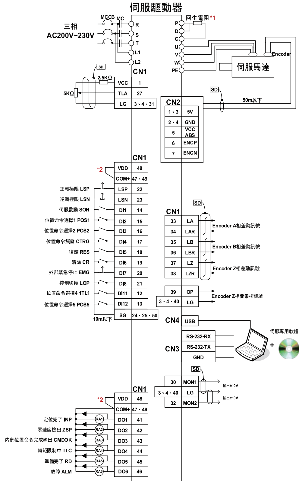
■ Pr Mode: 一軸內藏控制模式接線示意圖
