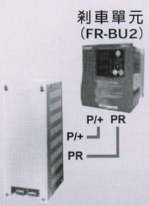
抵抗器單元 (FR-BR) 放電抵抗器 (GZG、GRZG) 可充分發揮變頻器的再生制動 能力。請視需要裝設。
