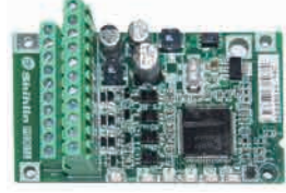
PG301L 速度回授卡 (支持差動式輸出)
